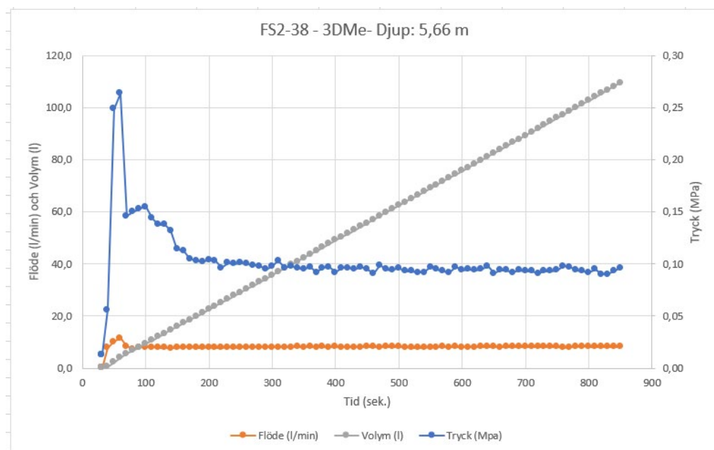
Figur 2 Sammanställning av injekteringsdata presenterad i graf-form. Aktuella grafer visar injekteringsdata för provpunkt FS2 38 på djupet 5,66 m
